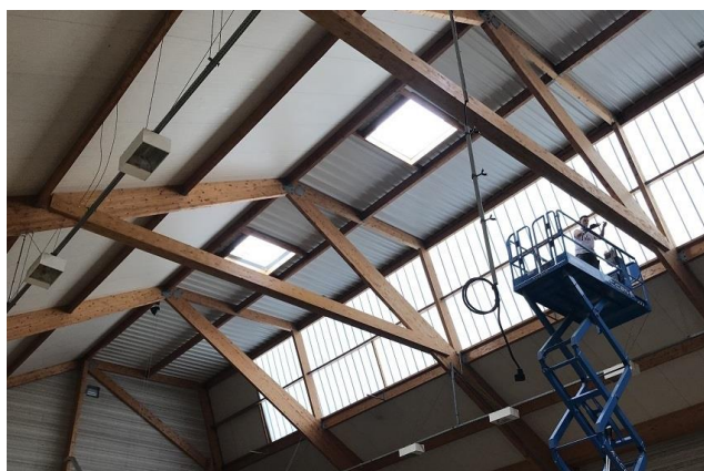
La charpente doit être réparée et renforcée. La toiture sera ensuite remplacée et la salle isolée.
